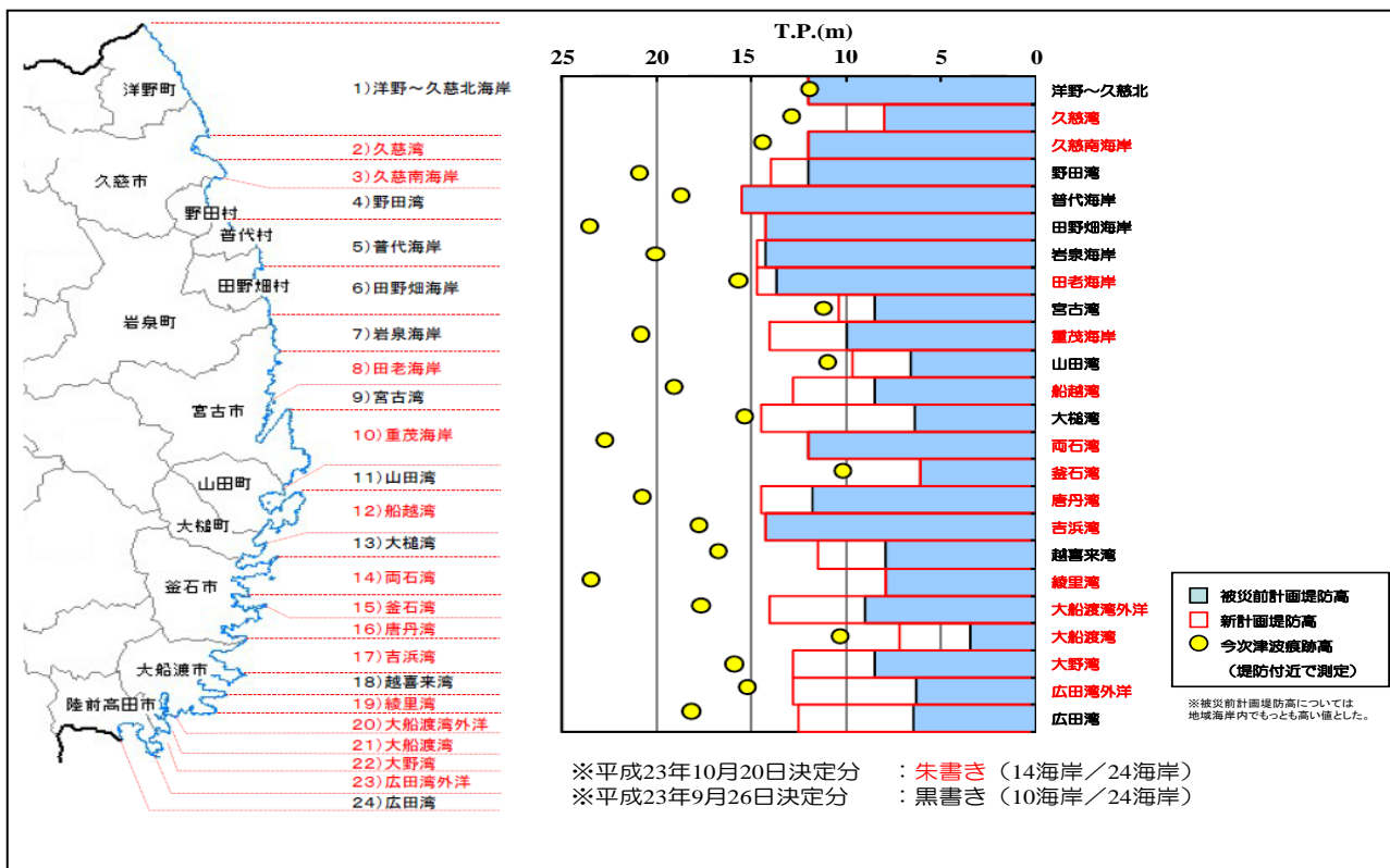
岩手県沿岸における海岸堤防高さの設定状況
