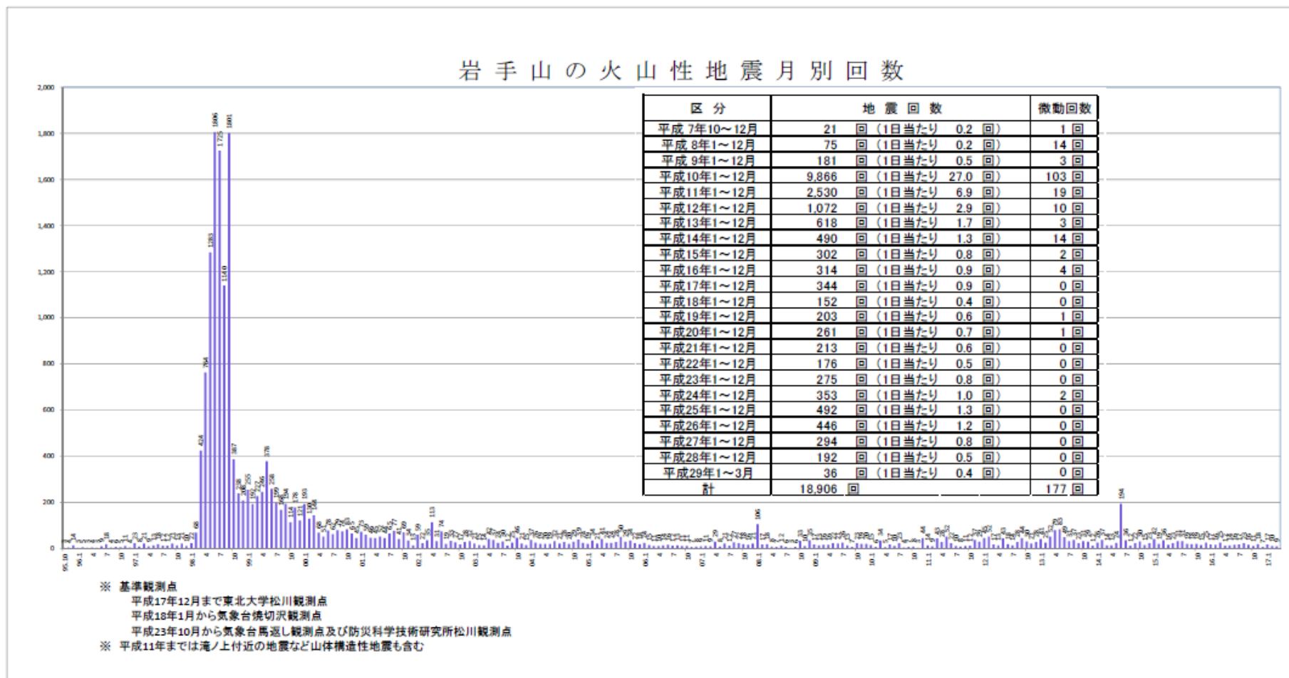
図3-2-1 岩手山の火山性地震月別回数
