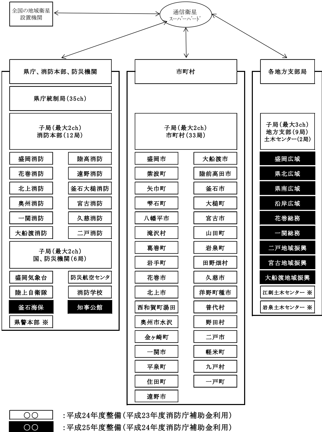
図3-3-1 防災行政情報通信ネットワーク構成図 H27.4.1現在
