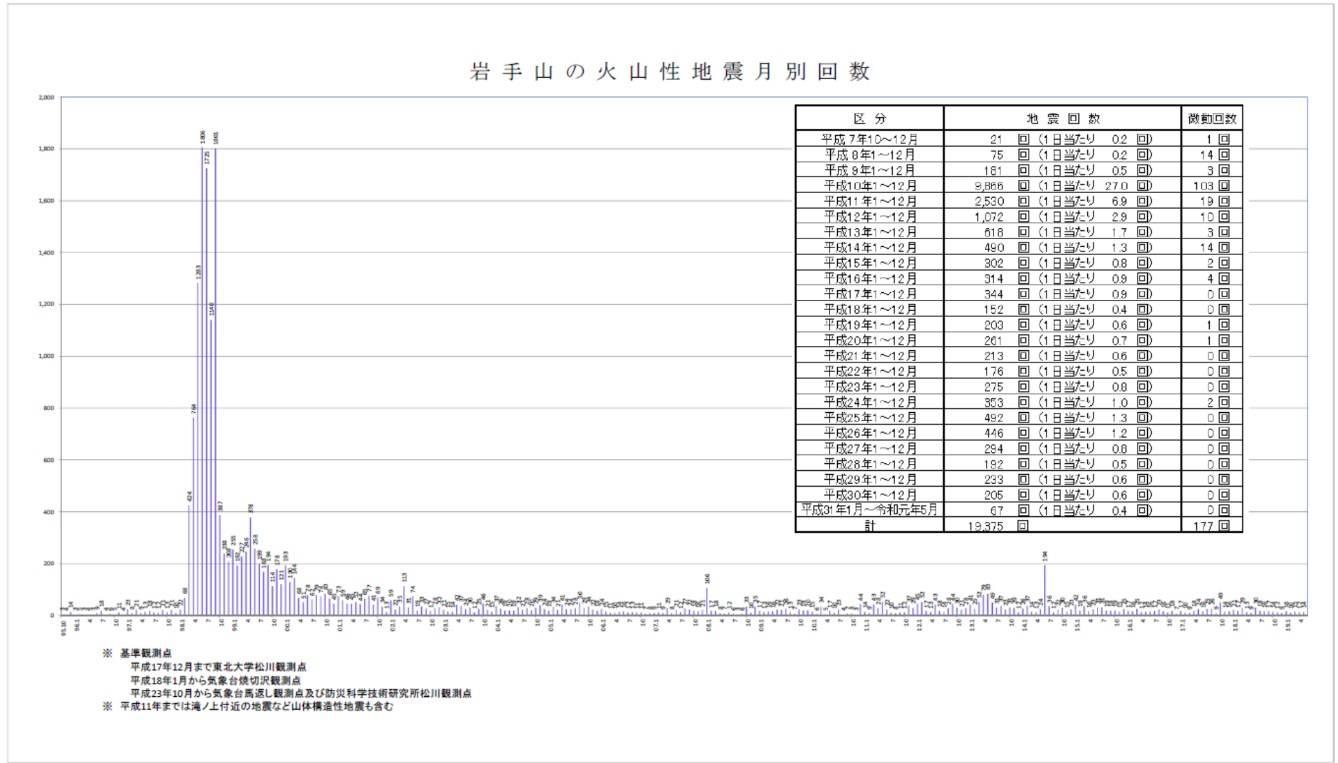
図3-2-1 岩手山の火山性地震月別回数
