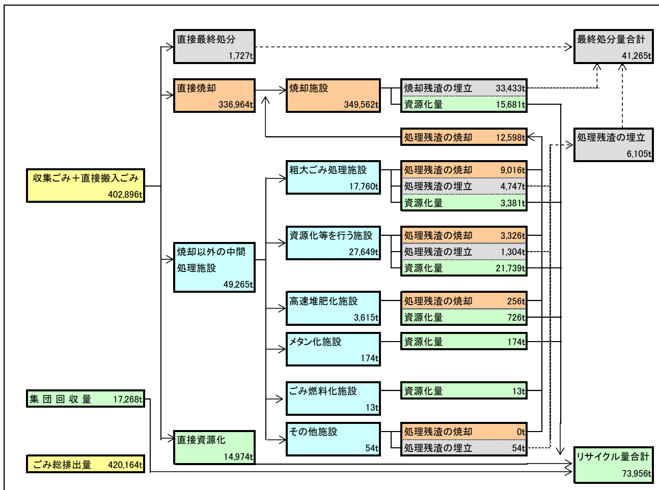
図-7 ごみ処理フロー図（令和元年度）
