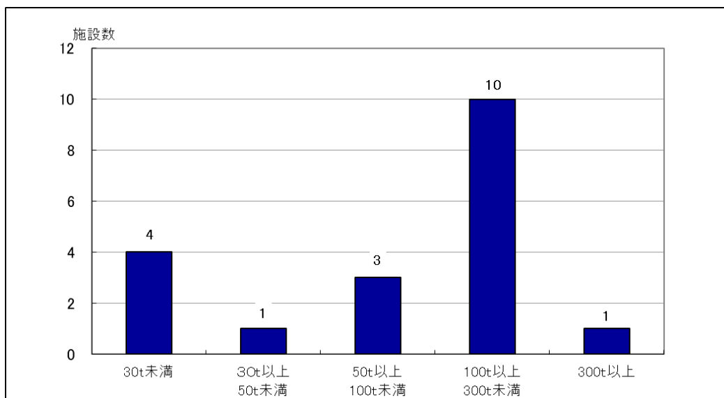
図-14 ごみ焼却施設の規模別施設数（令和元年度）
