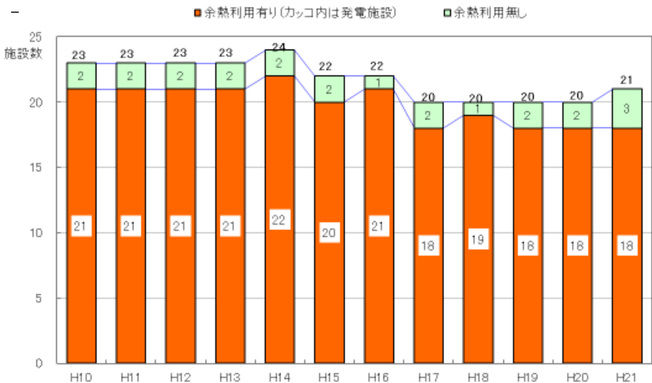
図－10 ごみ焼却施設の余熱利用の推移
