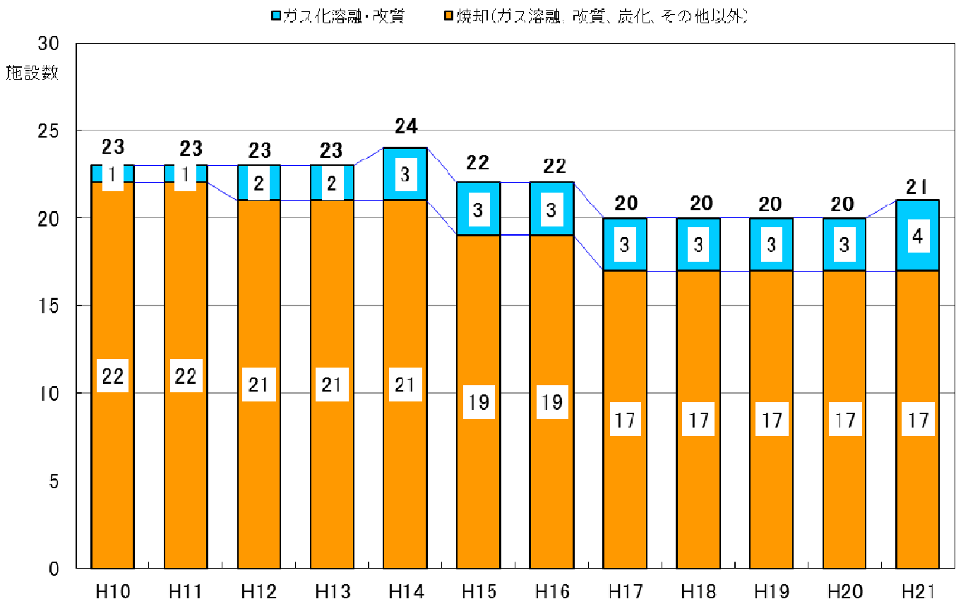
図－7 ごみ焼却施設の種類の別施設数の推移
