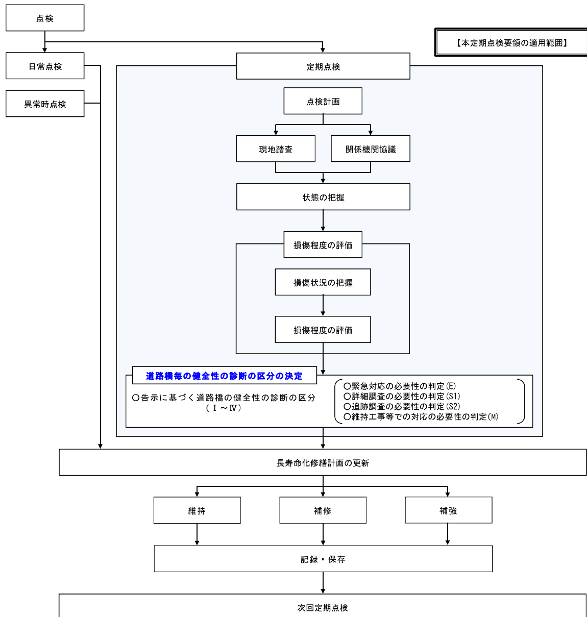
図－2. 3. 1 橋梁点検の流れ
