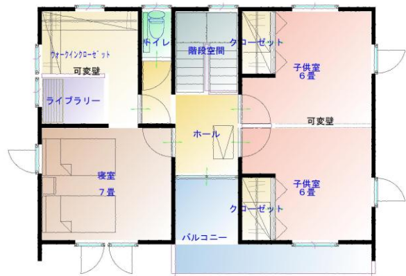
1/150 2階平面図
