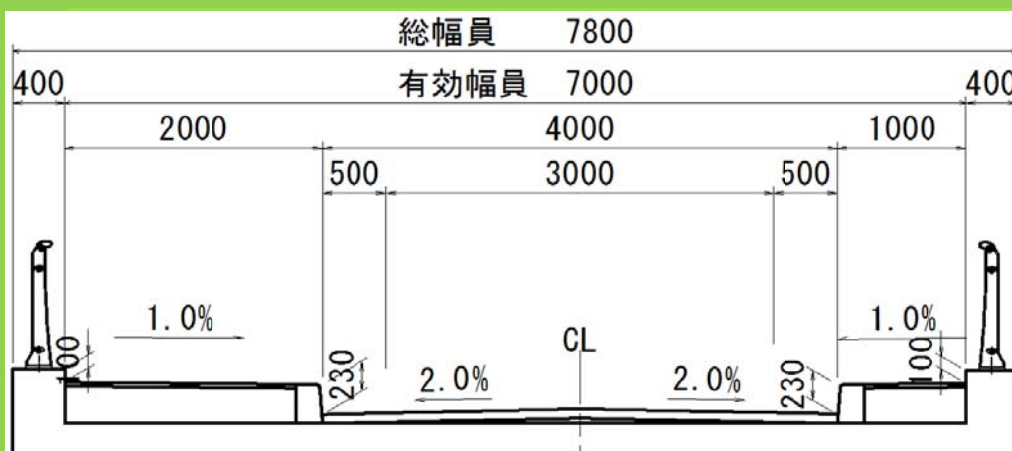
幅員構成：1車線+2（両側）歩道の標準横断図
