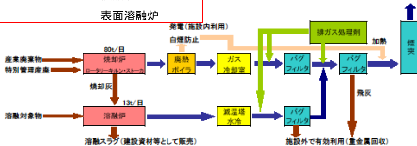
いわて第2クリーンセンター処理フロー
