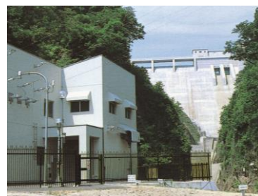
入畑発電所
