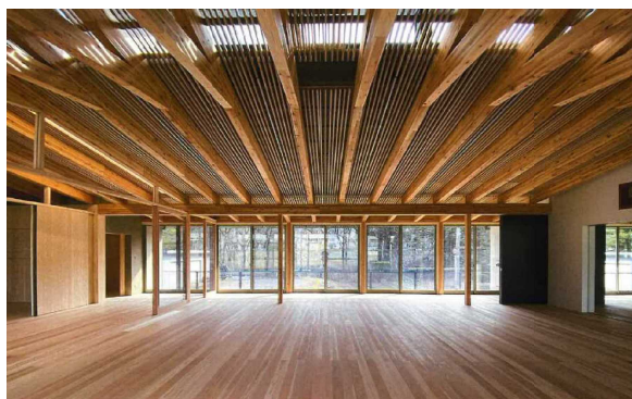
6 道の駅たのはた（田野畑村） 木造・木材使用量：208m 3 R3年度受賞
