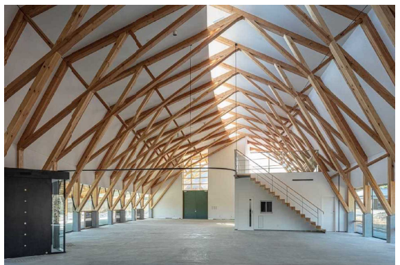
6 道の駅たのはた（田野畑村） 木造・木材使用量：208m 3 R3年度受賞
