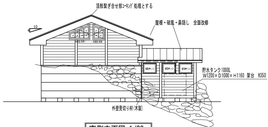
南側立面図 1/80
