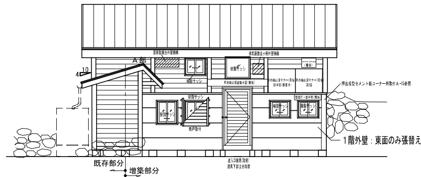
東側立面図 1/80
