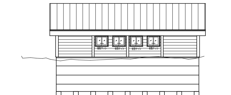
西側立面図 1/80
