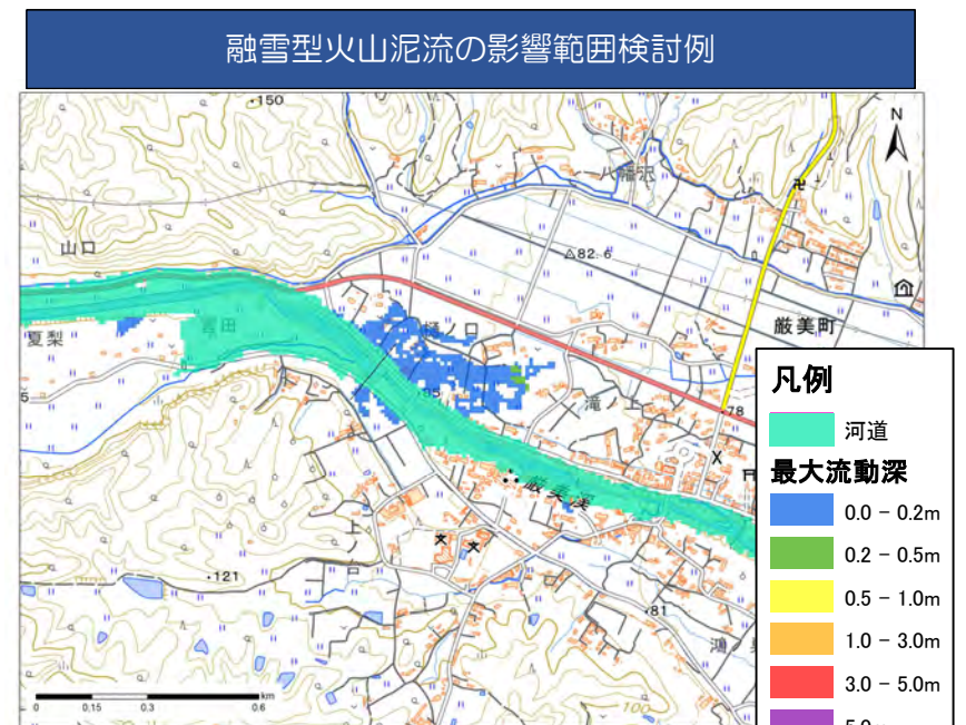
図4 磐井川(岩手県)の融雪型火山泥流計算例
