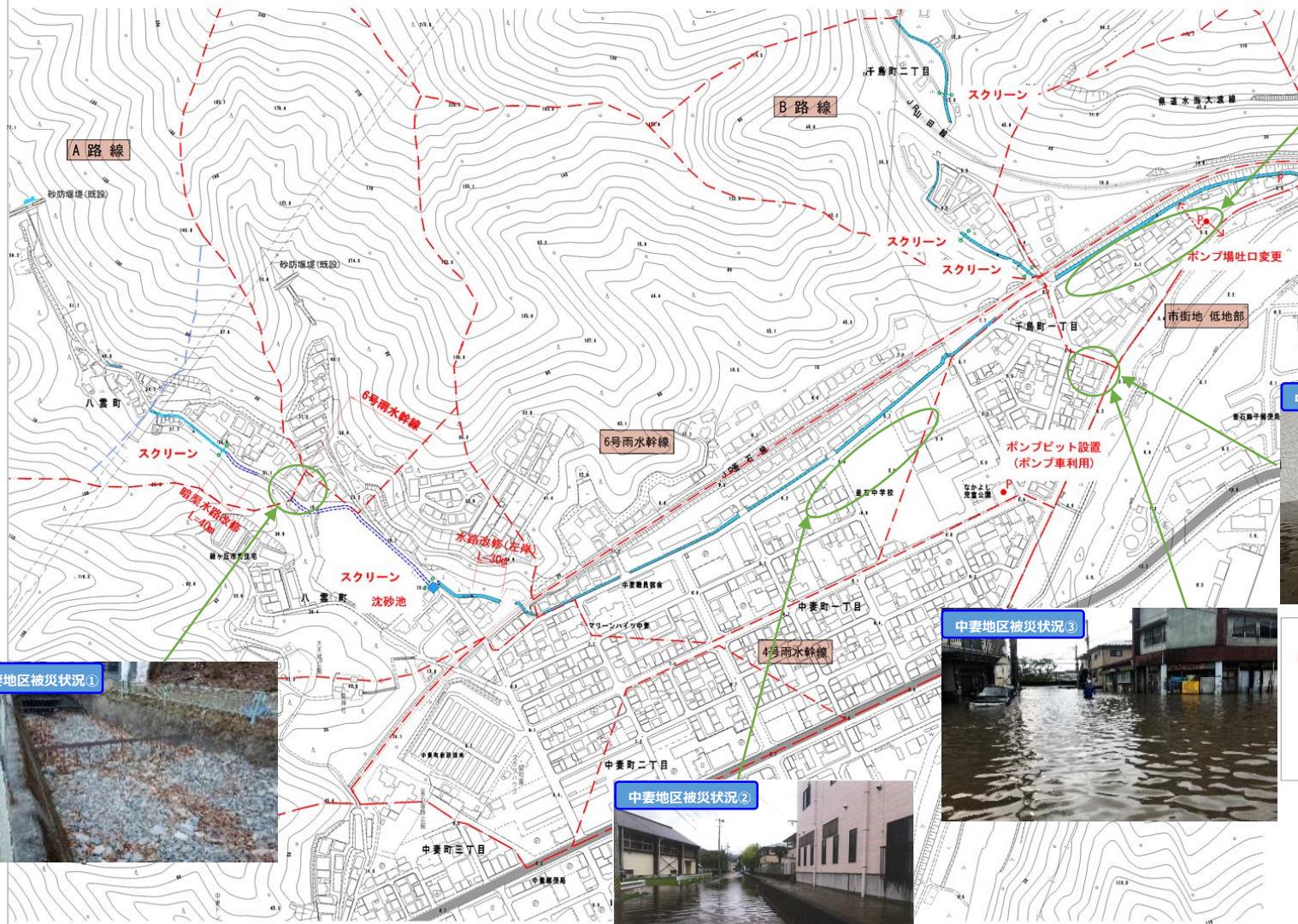
③中妻排水地区 対策検討図 ケース 1: S=1/4000 (1/2000)
