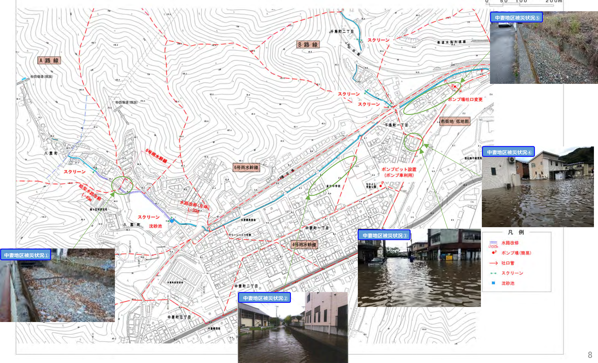
③中妻排水地区 対策検討図 S=1/4000 (1/2000) ケース 1:
