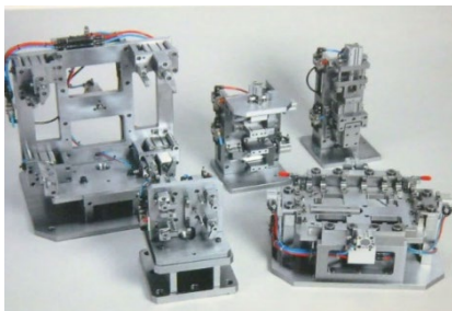
自社で開発～製作した治工具
