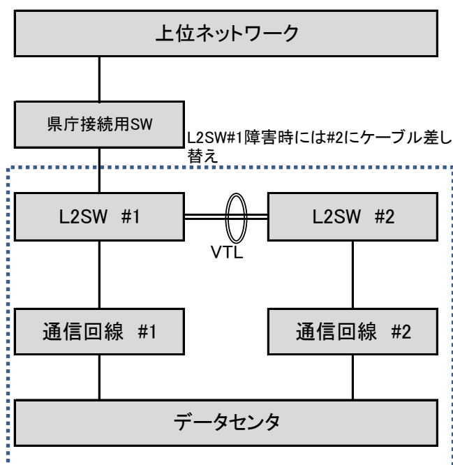
⑧中間サーバー連携セグメント用ネットワーク
