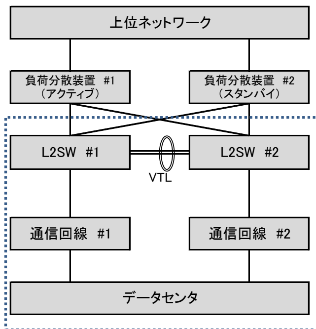
⑥総務事務システム負荷分散装置接続ネットワーク
