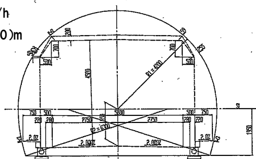
トンネル部標準断面図
