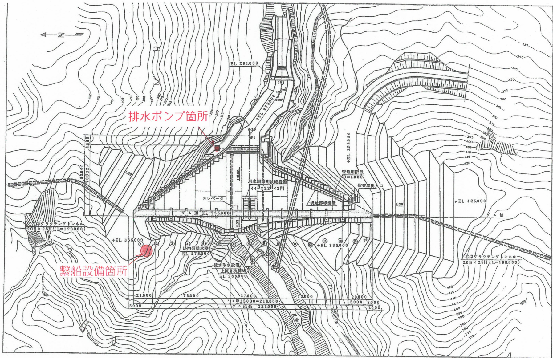
ダム平面
